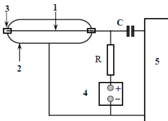
Рис. 1.1. Схема включения газового счетчика: 1- анод; 2 – катод; 3 – изолятор; 4- источник высокого напряжения; 5- блок регистрации; R – нагрузочное сопротивление; C - конденсатор
